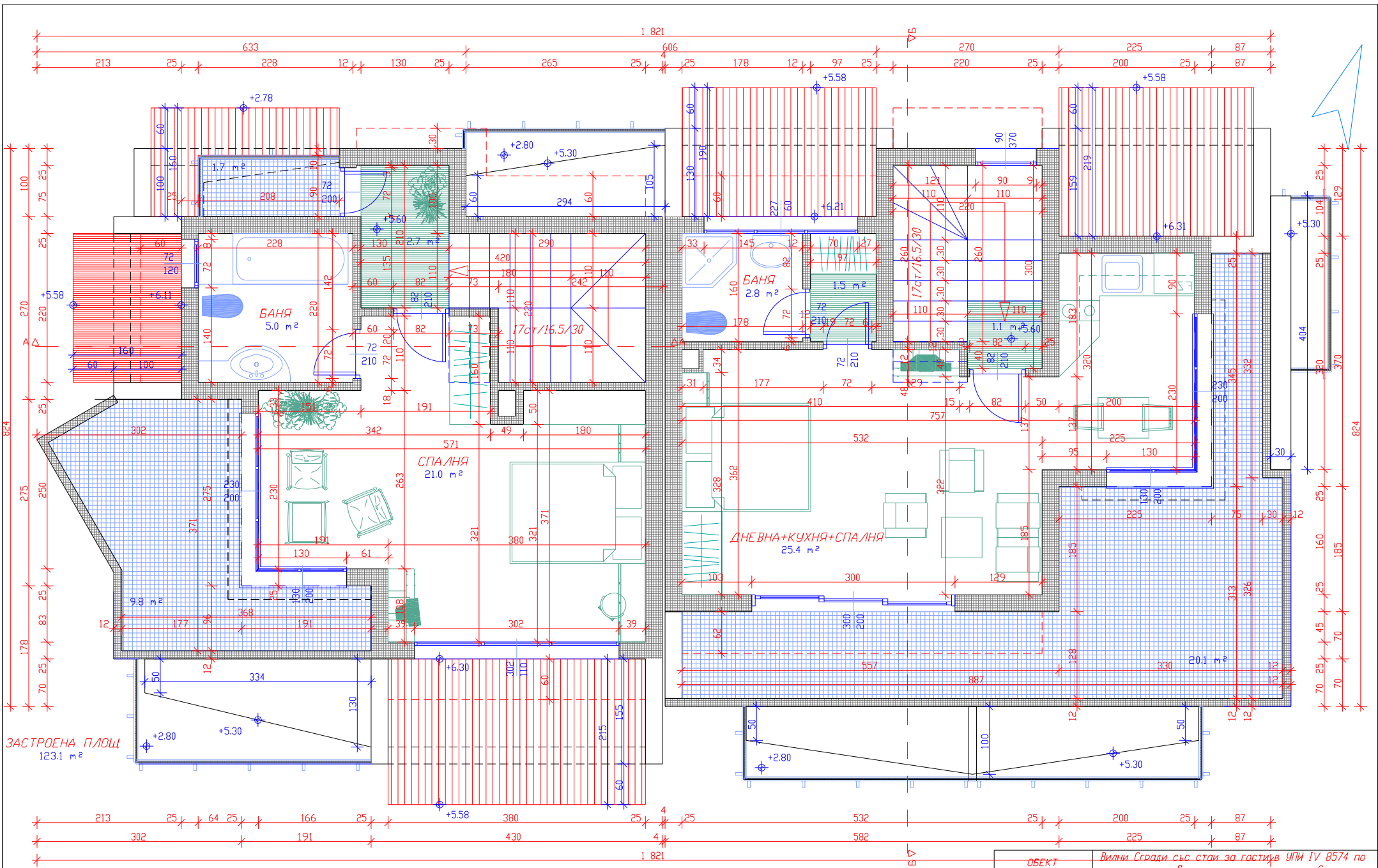
РАЗПРЕДЕЛЕНИЕ - КОТА +5.60 М 1:50
